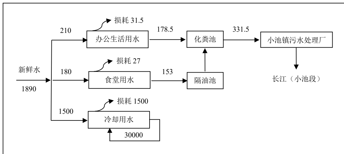
图 2-2 项目水平衡图 (单位: \text{m}^3/\text{a} )
