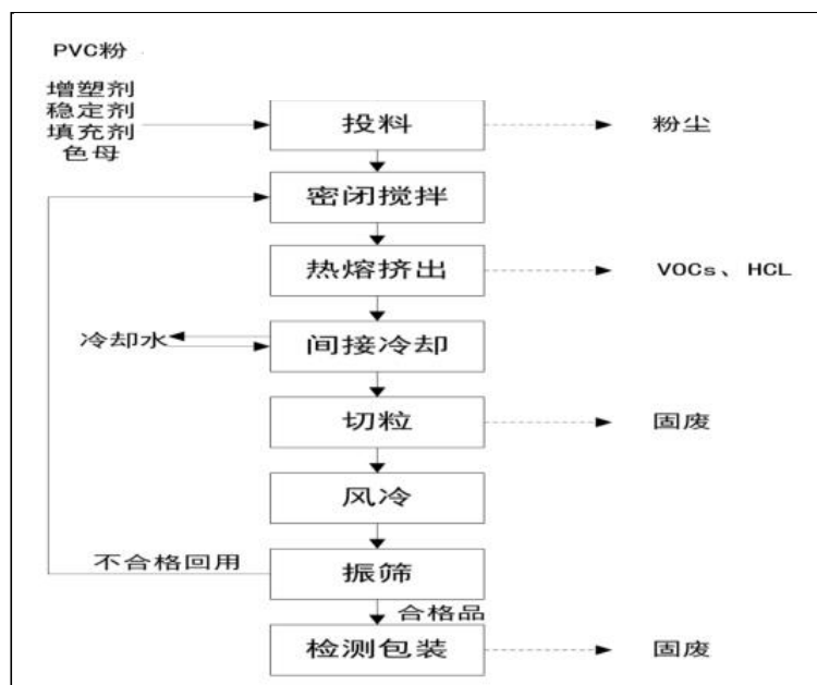
图 2-3 项目生产工艺流程及产污节点图
