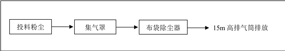
图 3-1 投料粉尘处理工艺流程图
