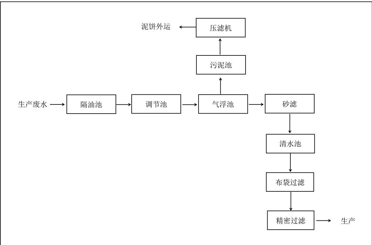
图 3-1 项目生产废水处理工艺流程图
